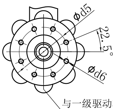
BA1~BA4法兰 A向
