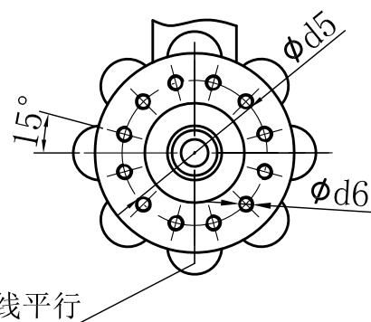
BA5法兰 A向
